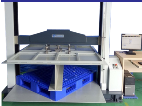
ĐỘ BỀN NÉN / COMPRESSION TEST
