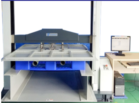
ĐỘ UỐN / BEND TEST
