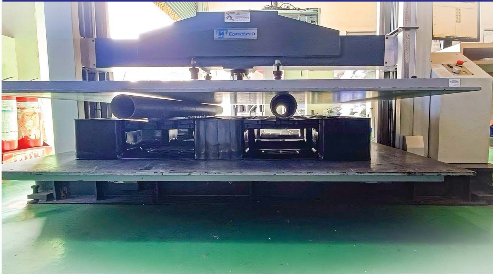
MÁY TEST PALLET / PALLET TEST MACHINE
